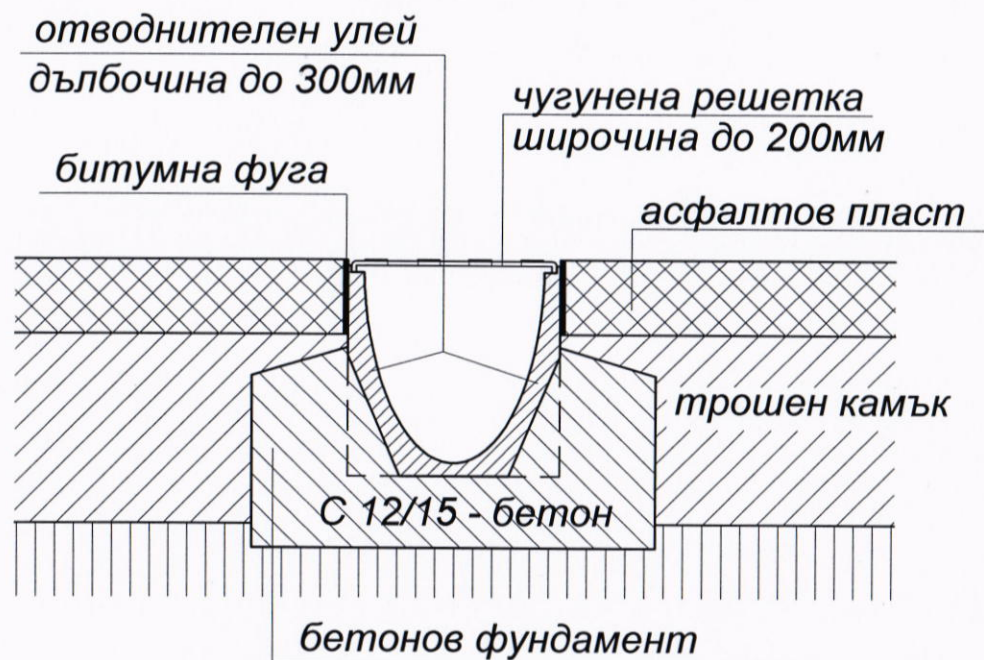
схема за монтаж
